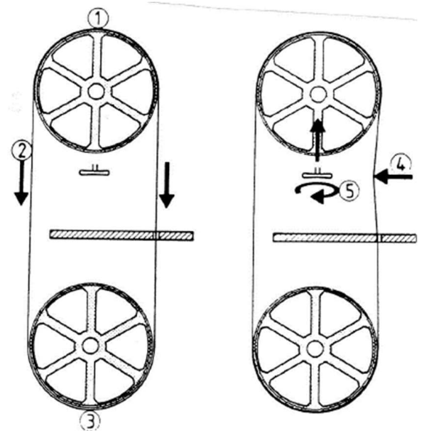
Bild 1: Auflegen und Aufspannen des Sägeblattes
